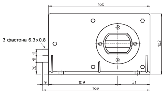
Вид спереди
