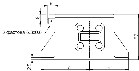
Вид спереди
