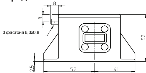
Вид спереди
