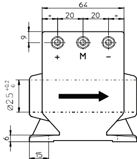
Вид спереди
